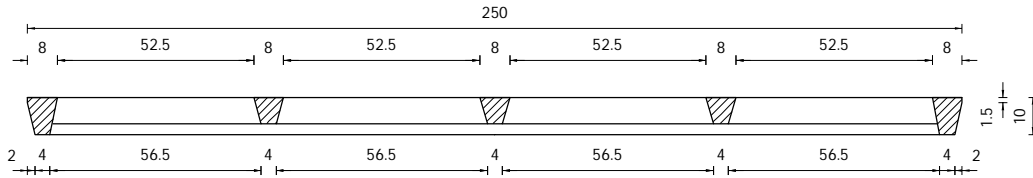
CORTE LATERAL
